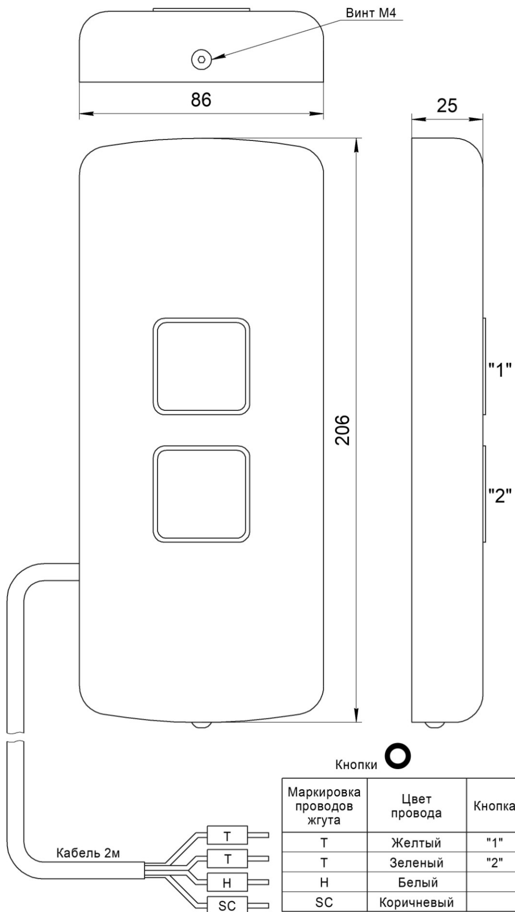
Рис.1 Внешний вид, габаритные и установочные размеры Вызывного поста ВП-2000-02
